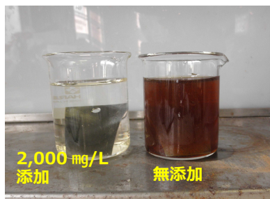
2,000 mg/L、軟鋼、1週間放置
